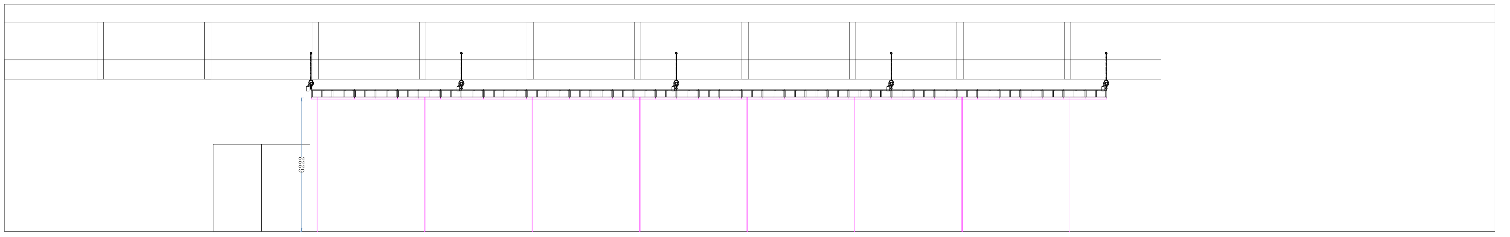
灯带侧视尺寸图6.5m (实际6.2m) *16根 小计: 104m
